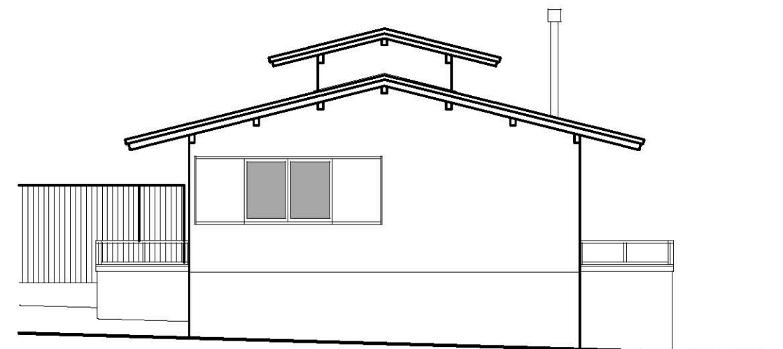
西立面図 S=1/00
