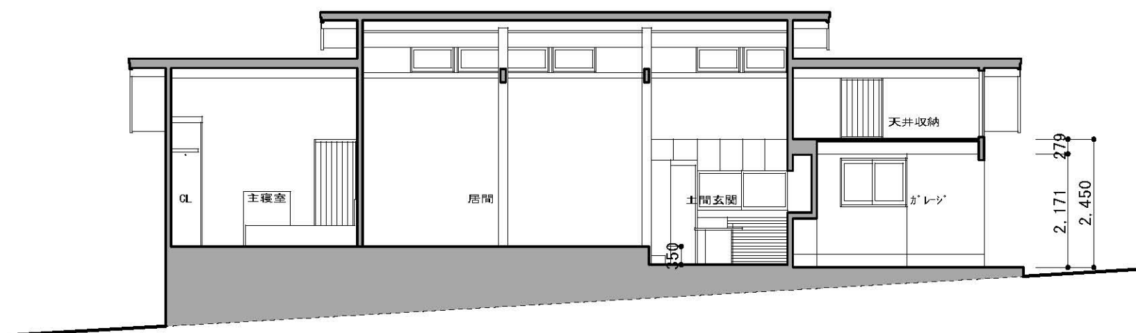
東西断面図 S=1/100
